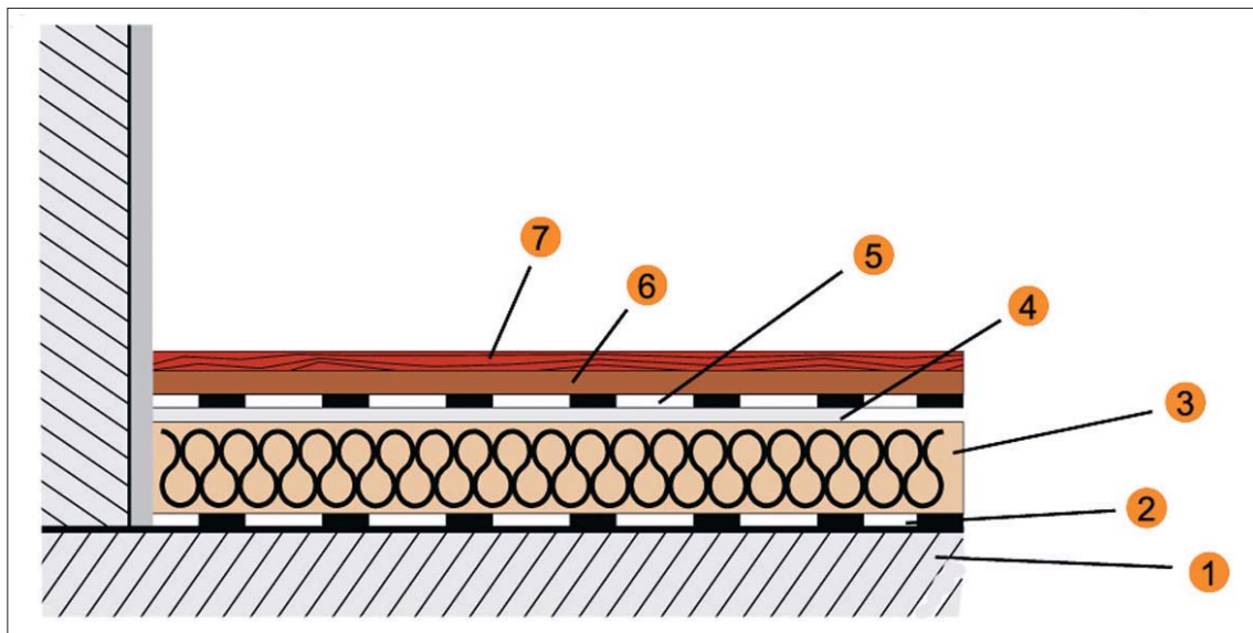
1 - strop, 2 - folia wodochronna, 3 - KONSTRUKTOR IP, 4 - wylewka betonowa, 5 - folia paroizolacyjna, 6 - KONSTRUKTOR FF, 7 - panele podłogowe
